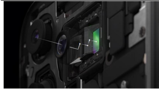
图表 8: 四重反射棱镜设计
