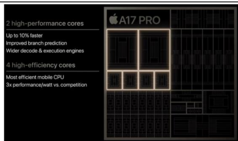
图表 5：A17Pro 芯片
